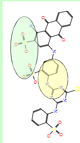
Cibacrone Blue F3G-A
