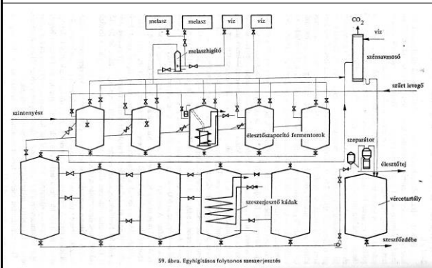
59. ábra. Egyhígítósú folytonos szeszgyártás
