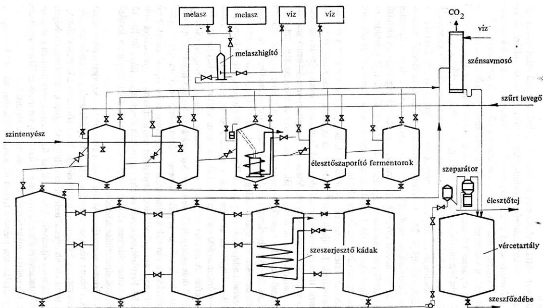
59. ábra. Egyhígítósos folytonos szeszferjesztés
