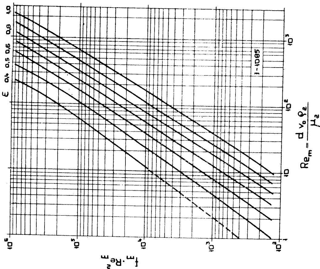
12. ábra Töltött oszlopok f_m \cdot Re_m^2 - Re_m diagram
