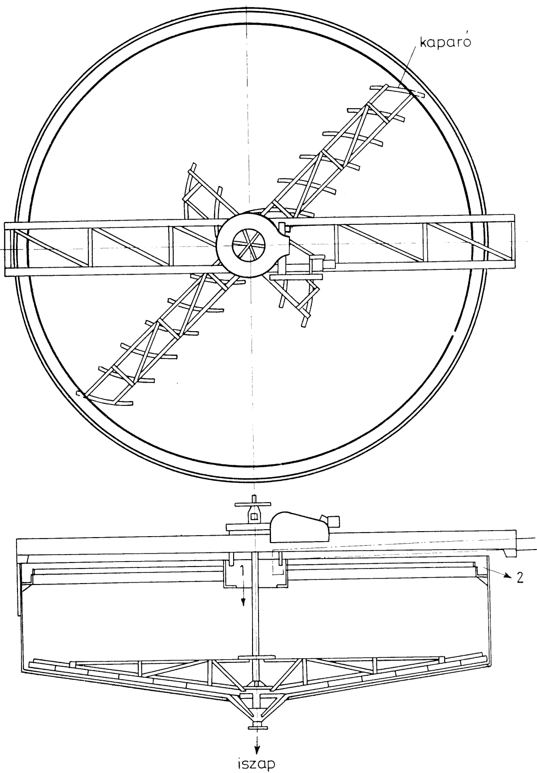
4.17. ábra Dorr-ülepítő
