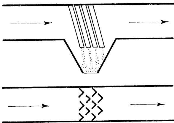
4.11. ábra Írányeltéritésen alapuló ülepítő
