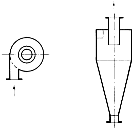
4.7. ábra Ciklon
